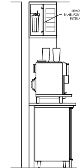
SECTION SCALE: 3/4"=1'-0"
